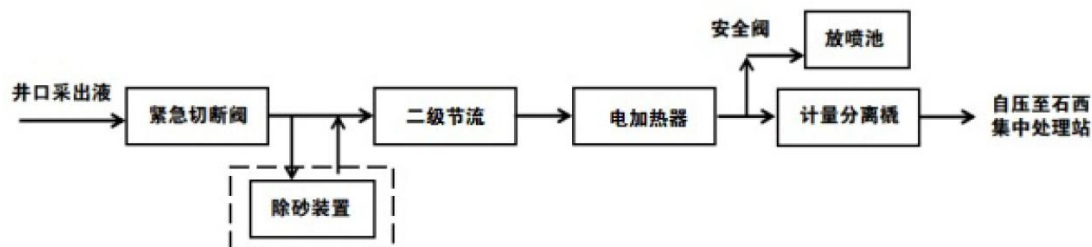
图 3.3-3 集输工艺流程示意图
