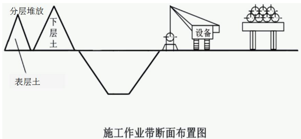
图 3.2-2 一般地段管道施工方式断面示意图
